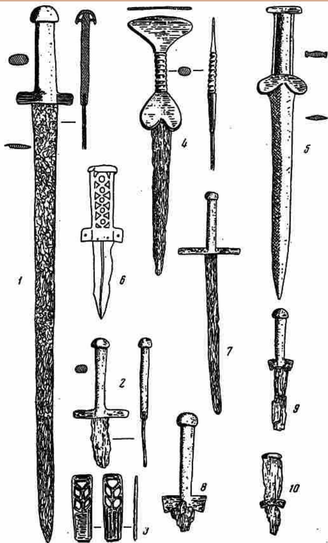
Металлическое оружие скифов: 1 — железный меч из-под Киева; 2 — железный кинжал; 3 — бронзовая рукоятка железного кинжала; 4 — железный кинжал; 5 — бронзовый кинжал; 6 и 7 — кинжалы (Венгрия); 8—10 — железные кинжалы (Северный Кавказ)
